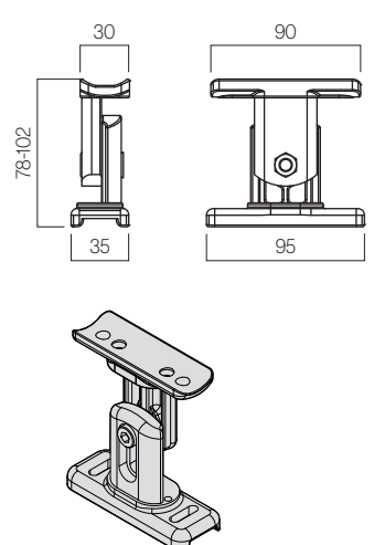
Support de guidage réglable
