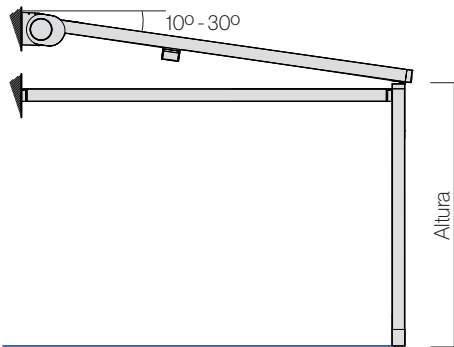
Vista lateral
