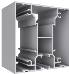
Trave guida 125x125 mm
