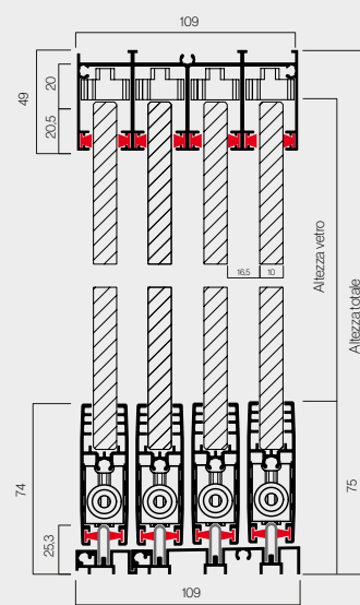
Sezione con 4 ante
