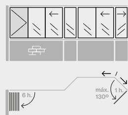
Terrazza quadrangolare aperta su due lati. Angolare da 135°
