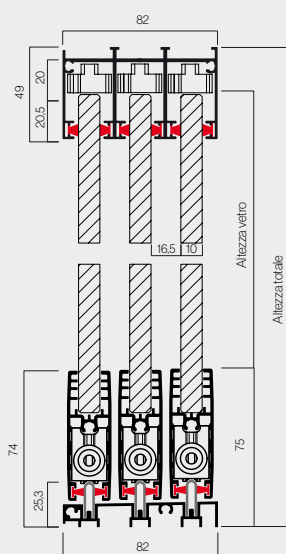
Sezione con 3 ante
