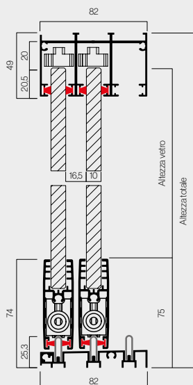
Sezione con 2 ante
