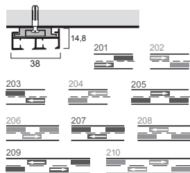
Binario 2 vie
