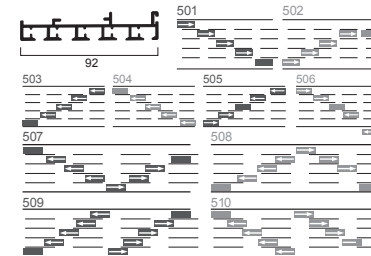
Binario 5 vie
