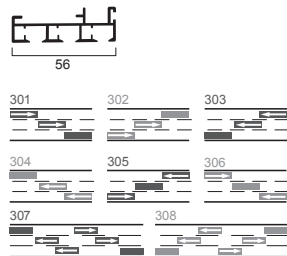
Binario 3 vie
